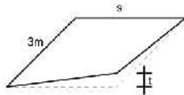
Fig. 5.2.14 - Sghembo ammissibile
