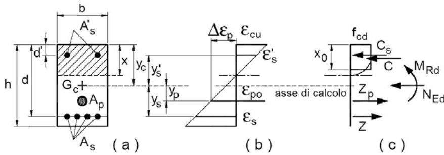
Fig. 4.1.4 – Sezione pressoinflessa
