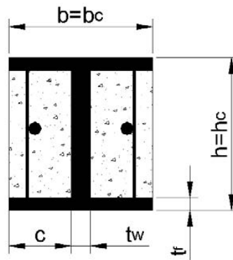
Fig. 7.6.1 - Rapporti dimensionali
