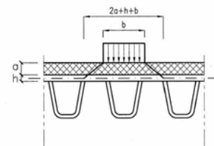
Fig. 5.1.3b - Diffusione dei carichi concentrati negli impalcato a piastra ortotropa
