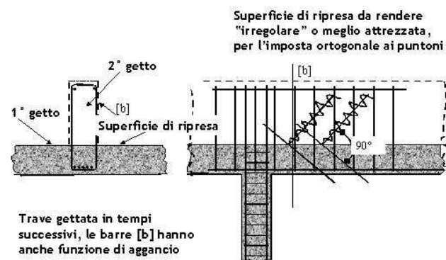
Figura 5-10: Ripresa di getto su travi di spessore elevato
