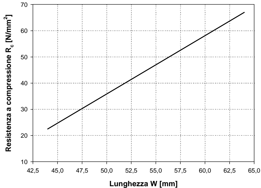
Figura 12-5: Andamento esemplificativo della correlazione tra lunghezza [W] e resistenza a compressione [Rc].
