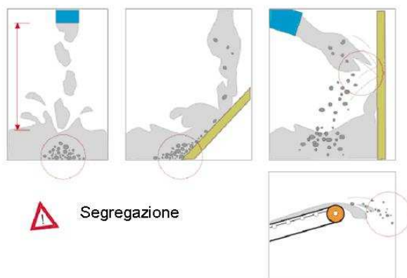
Figura 5-5: Errori nella posa in opera del calcestruzzo
